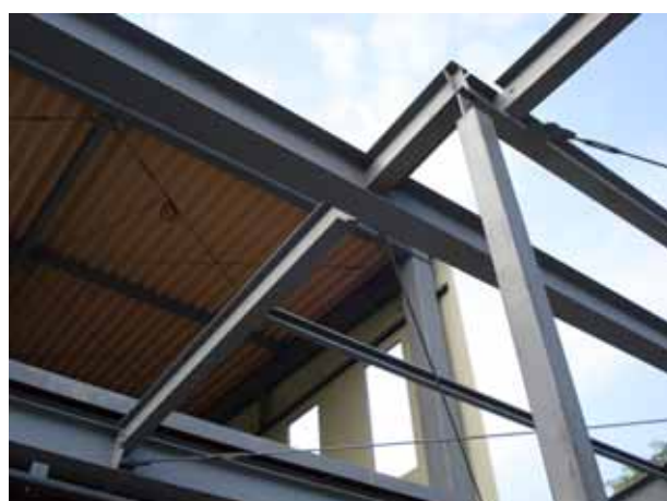
鉄骨組立
